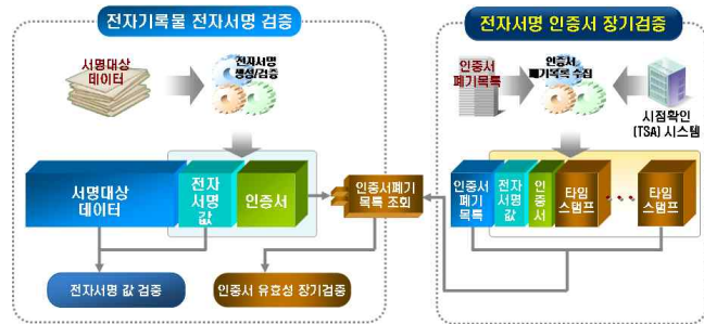
그림 5 - 전자서명 인증서 장기검증
