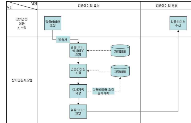
그림 17 - 검증데이터 요청 절차
