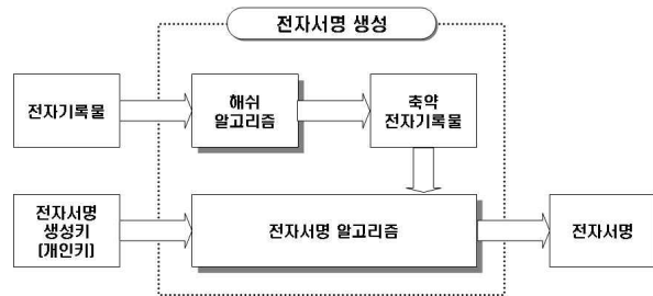
그림 1 - 전자서명 생성 과정
