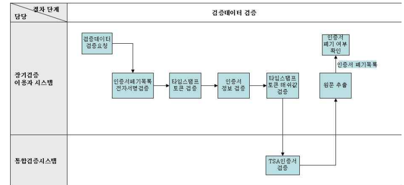
그림 18 - 장기검증데이터 검증의 세부처리 절차
