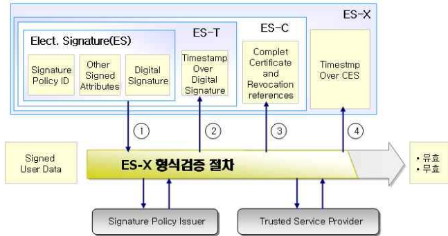
그림 19 - ES-X 형식 검증 절차
