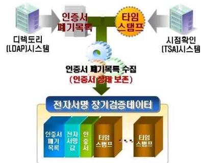
그림 6 - 장기검증데이터의 생성 방법
