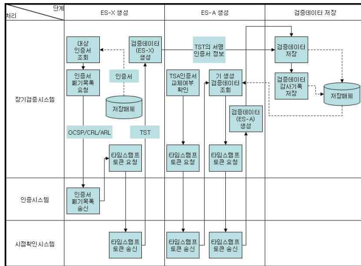
그림 16 - 장기검증데이터 생성을 위한 세부절차
