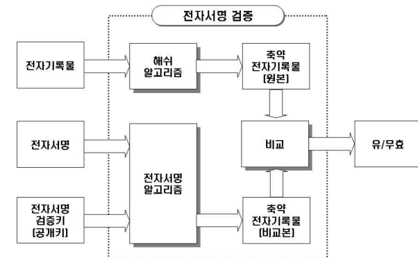
그림 2 - 전자서명 검증 과정
