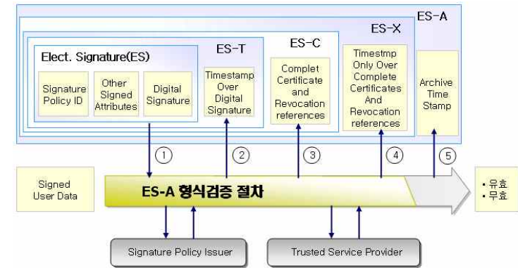
그림 20 - ES-A 검증 절차
