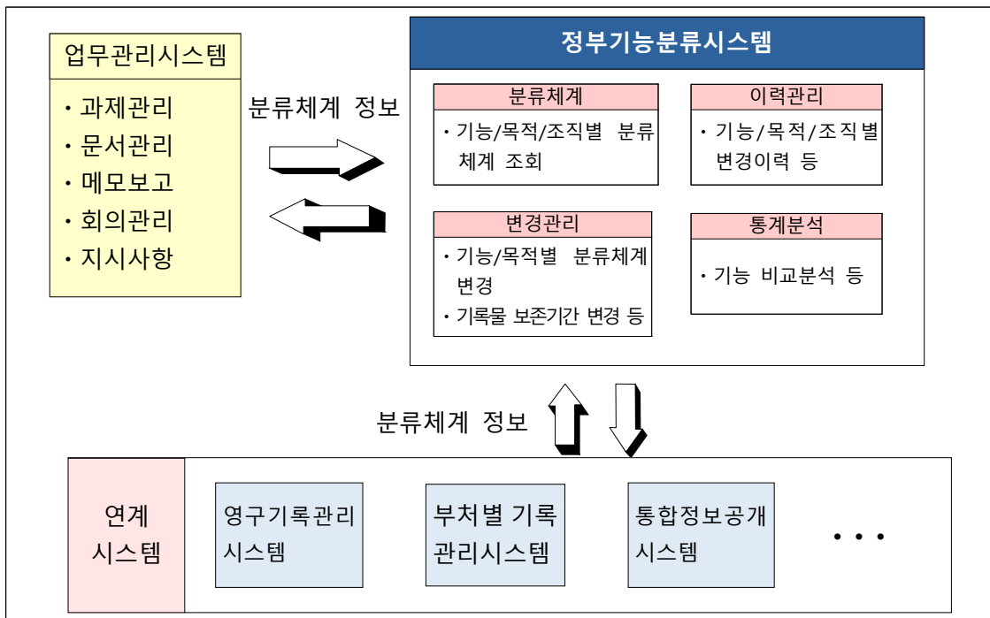
그림 1 - 정부기능분류시스템 연계도
