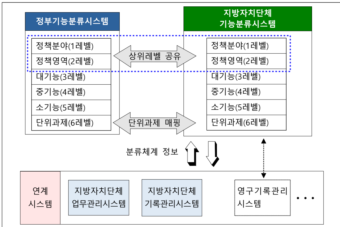
그림 2 - 지방기능분류시스템 연계도
