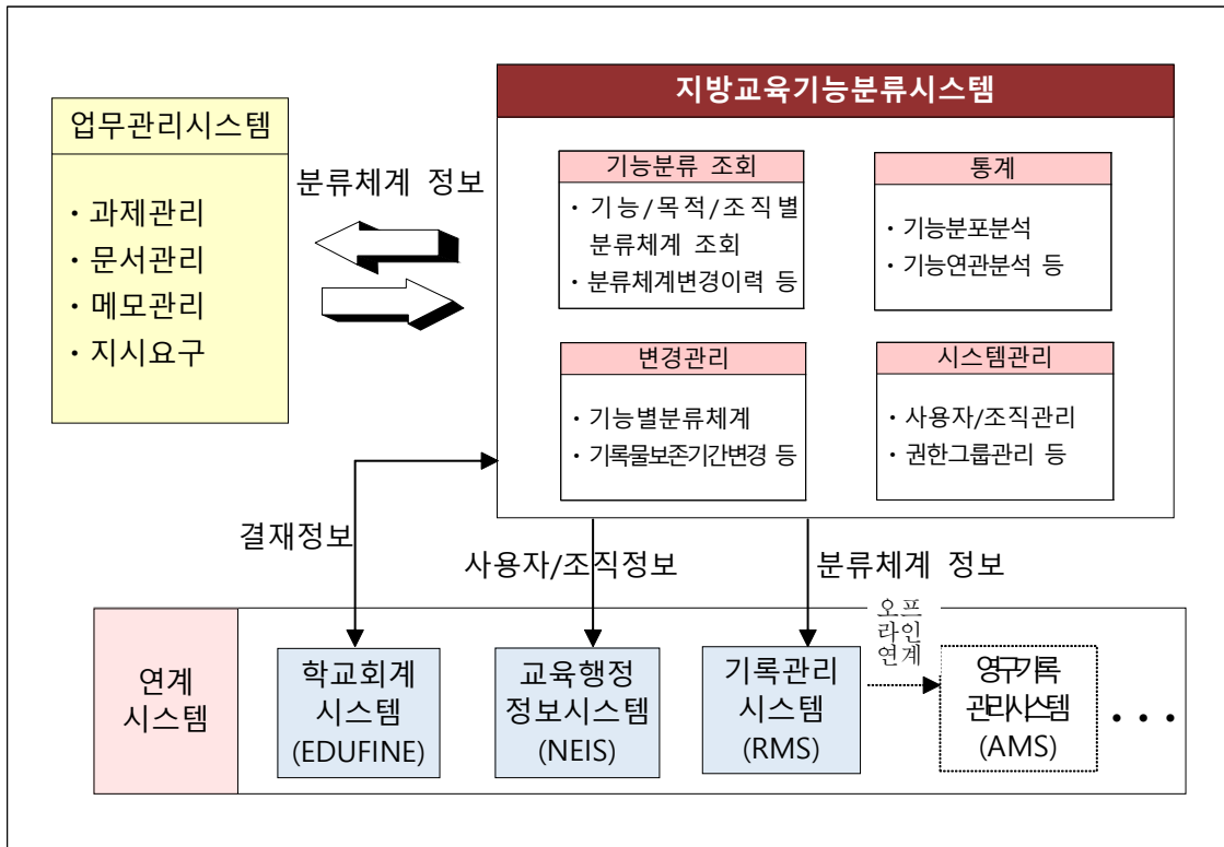
그림 3 - 지방교육기능분류시스템 연계도
